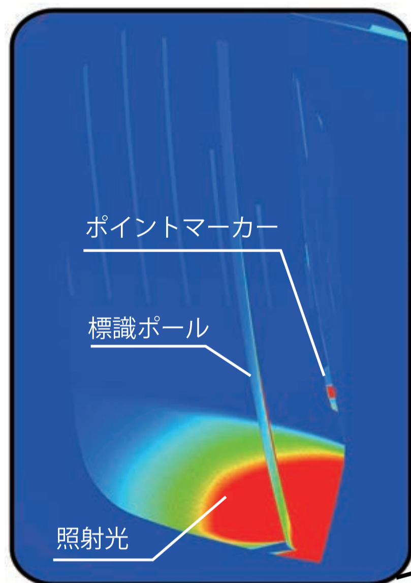
ミラー視点光学解析結果 青→赤になるにつれ明るい
